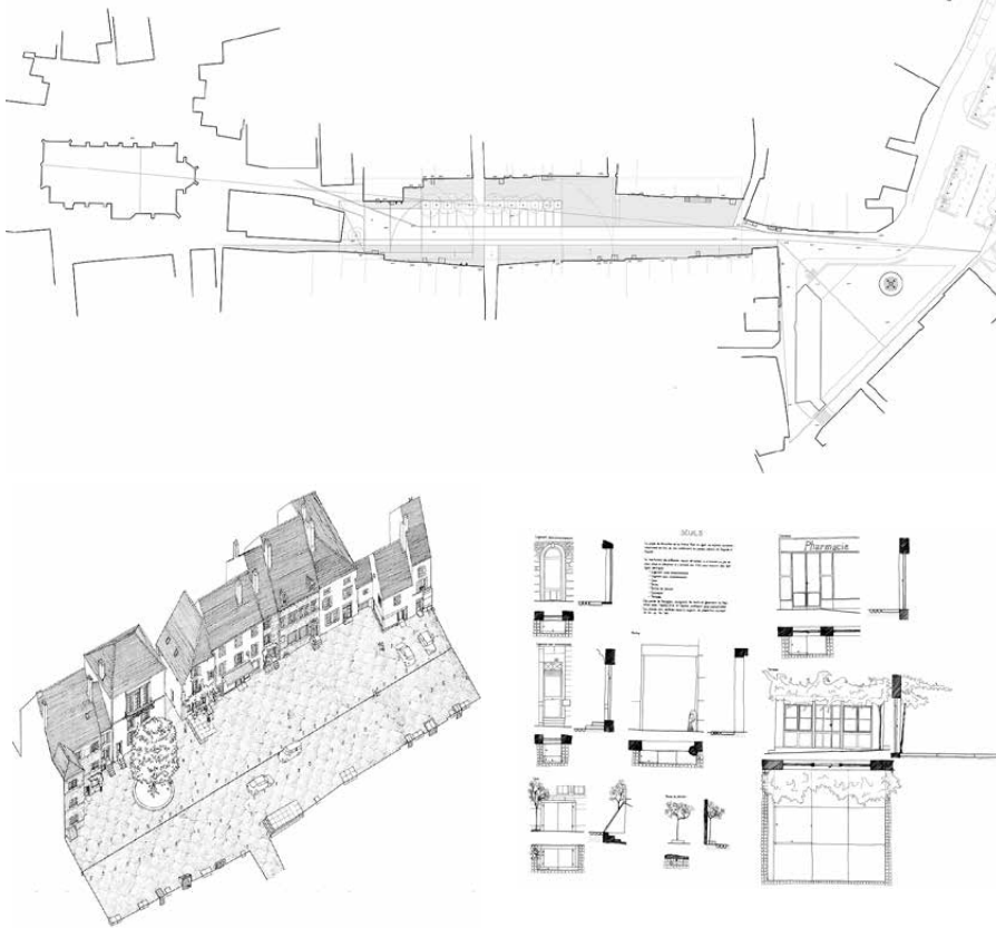
Plan du projet pour la Grande-Rue, axonométrie et détails des seuils réalisés par les étudiants pendant le séminaire 2020. (© BQ+A.)
